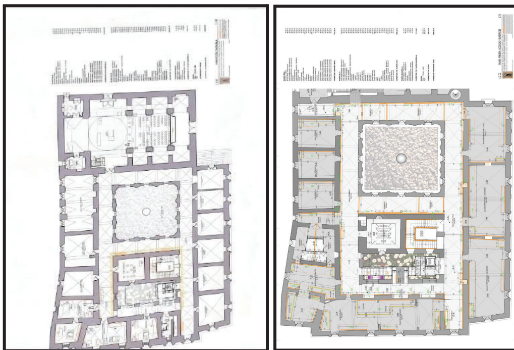
Planos planta baja y planta primera donde están ubicados los espacios que utiliza el COD
